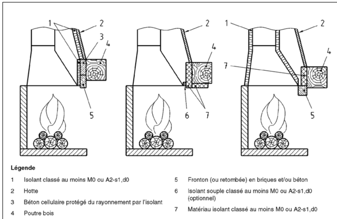
Figure A.1 - Exemple de protection thermique de la poutre de l'âtre
