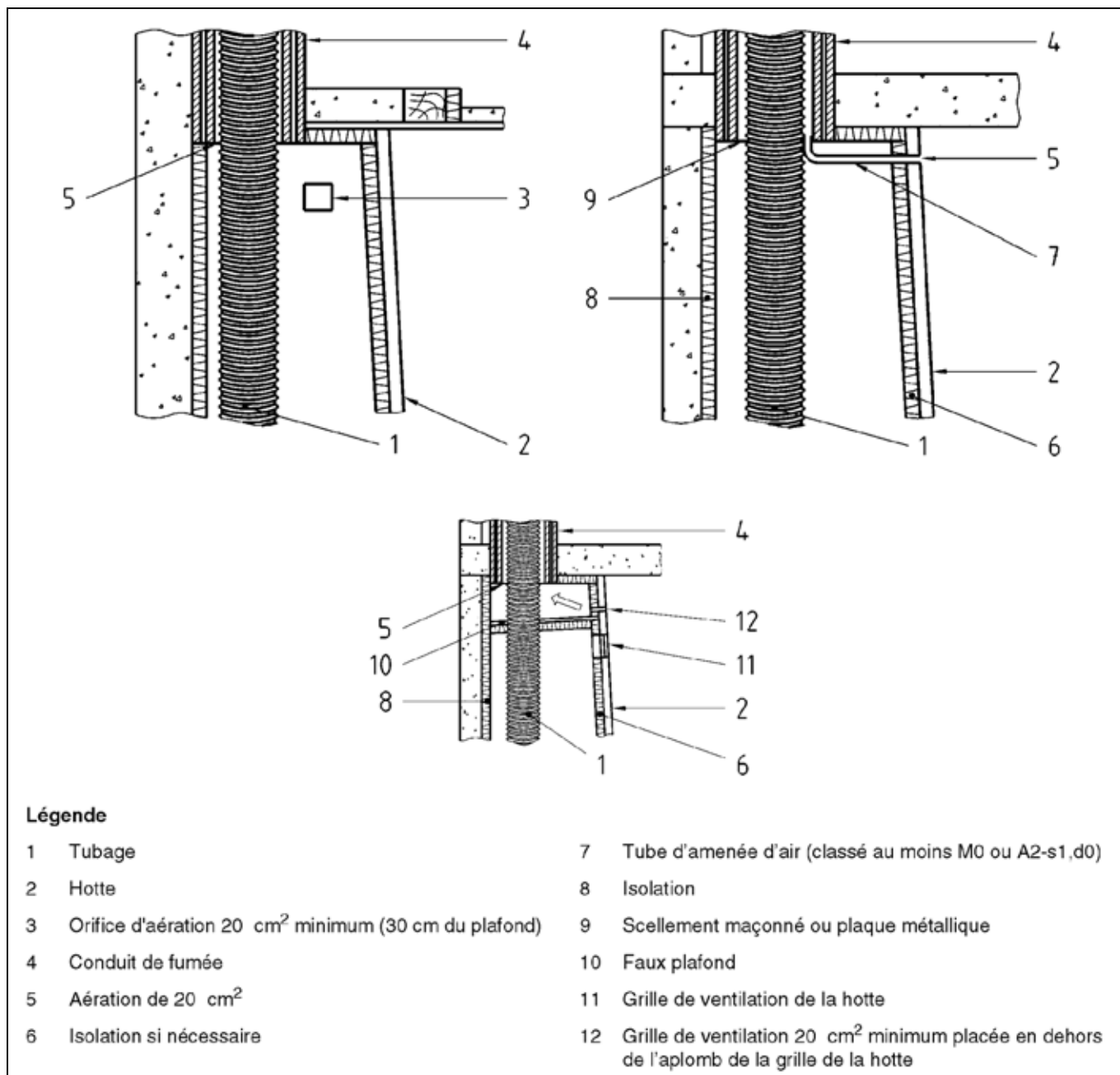
Figure 14 - Exemples de ventilation ou d'aération de l'espace annulaire
