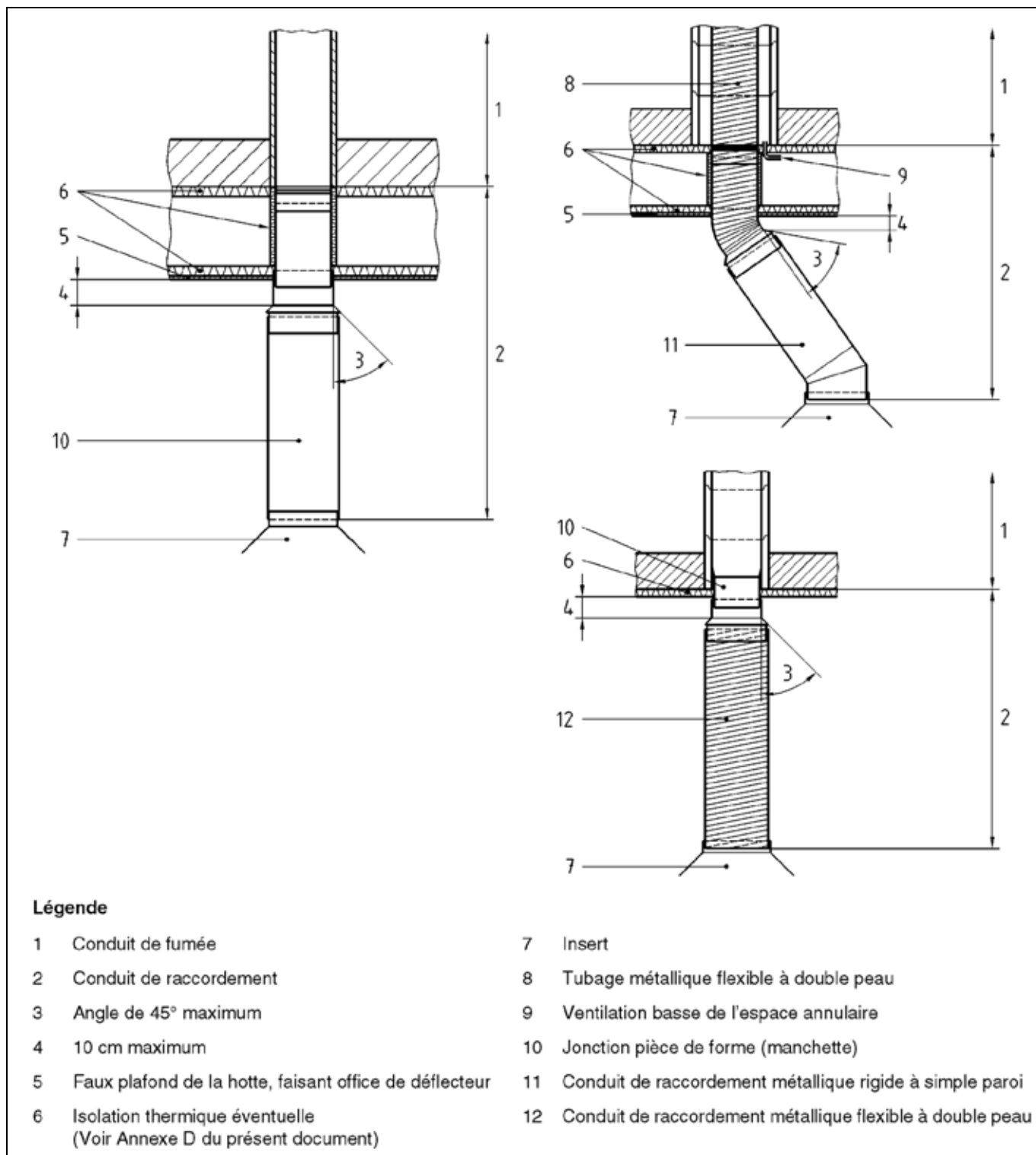
Figure 10 - Exemples d'une variation de section sur un conduit de raccordement
