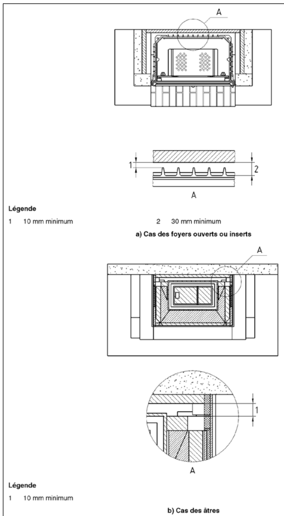
Figure 2 - Protection des parois des locaux servant d'adossement à la cheminée
