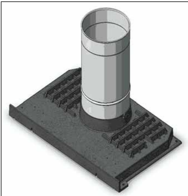
Figure 11 - Exemple de jonction du conduit de raccordement sur la buse (mâle)
