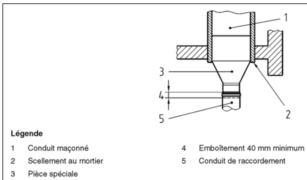
Figure 3 - Raccordement avec élément spécial
