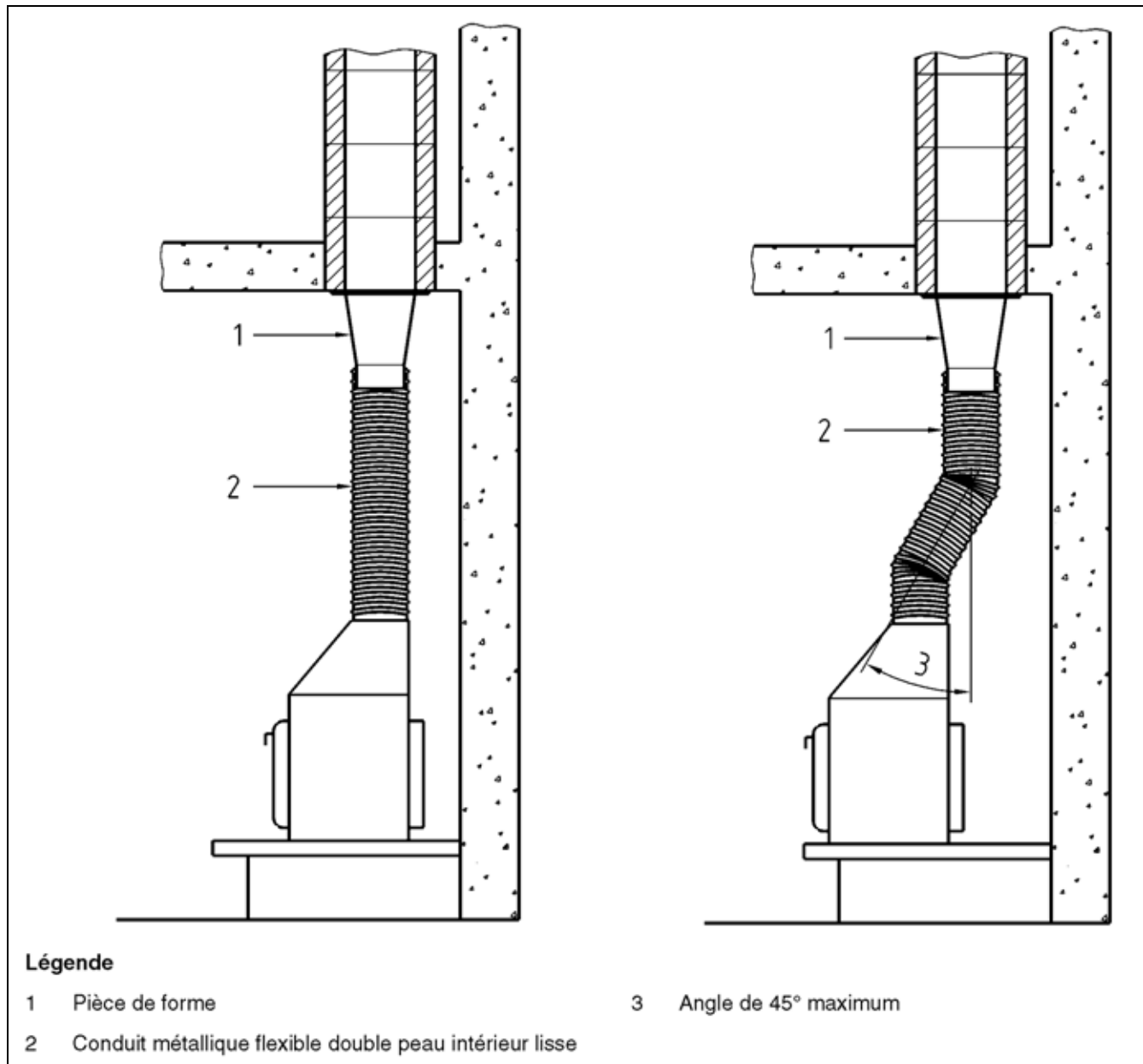
Figure 5 - Exemples de jonction d'un conduit de raccordement métallique flexible double peau avec un conduit de fumée maçonné
