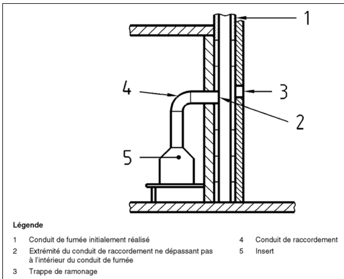
Figure 7 - Jonction sur un conduit maçonné en situation extérieure partant du sol (exemple de solution)
