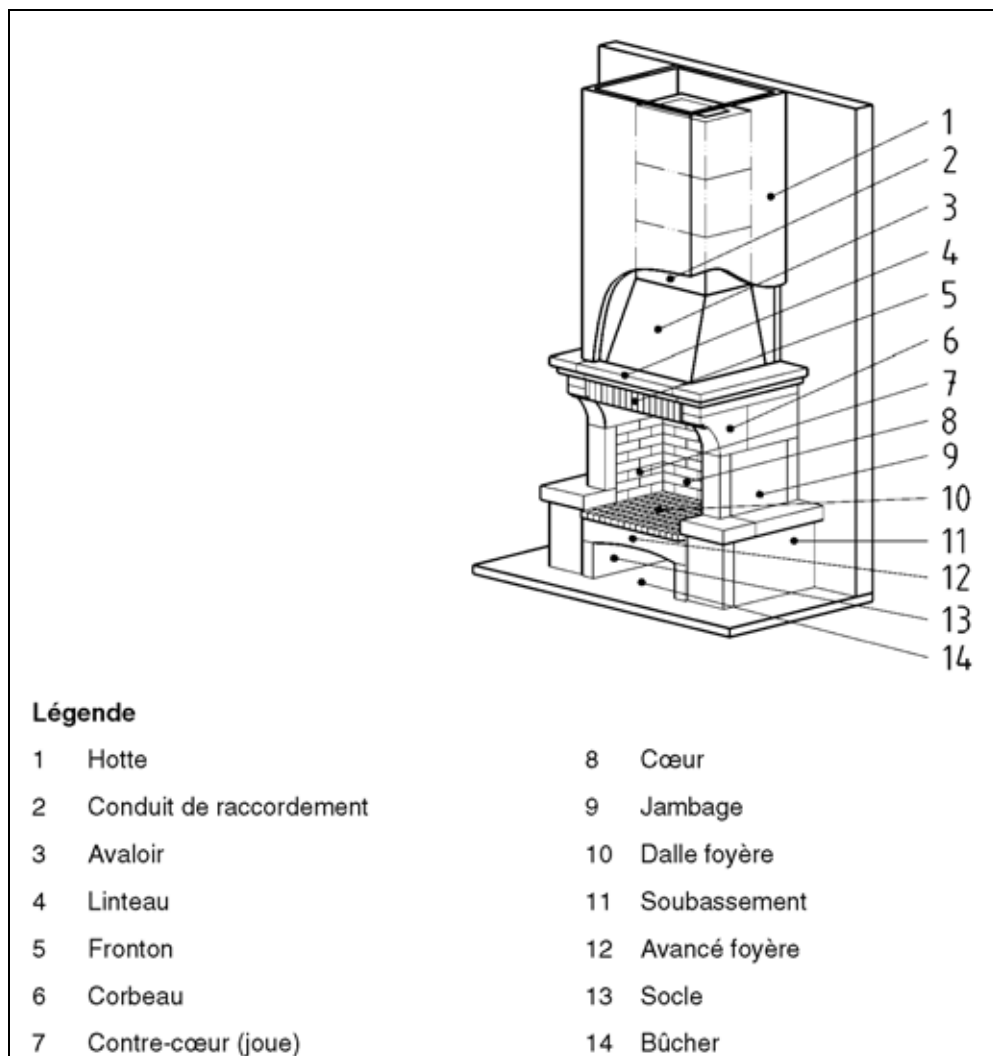
Figure 1 - Dénomination des diverses parties de l'évacuation des fumées
