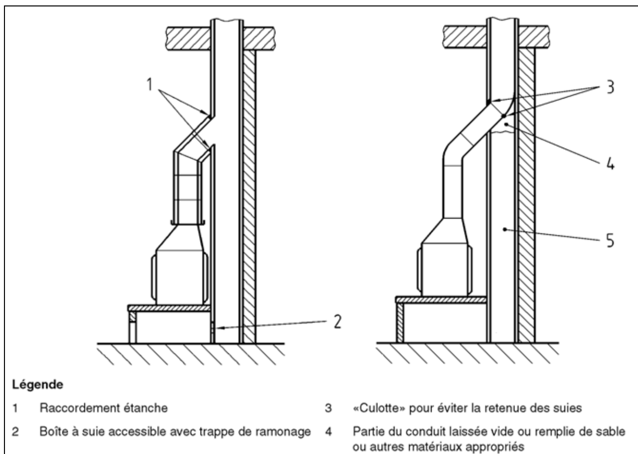
Figure 6 - Jonction d'un conduit de fumée maçonné en situation intérieure partant du sol
