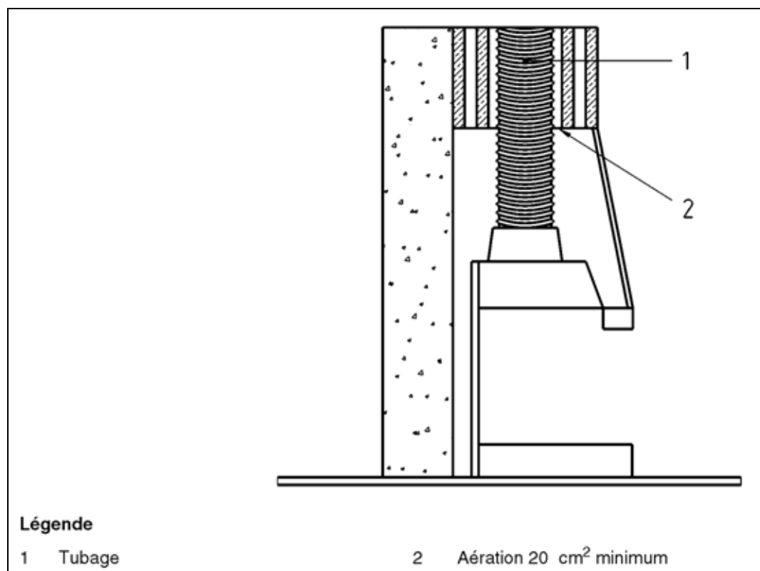
Figure 13 - Exemple de raccordement direct sur un tubage
