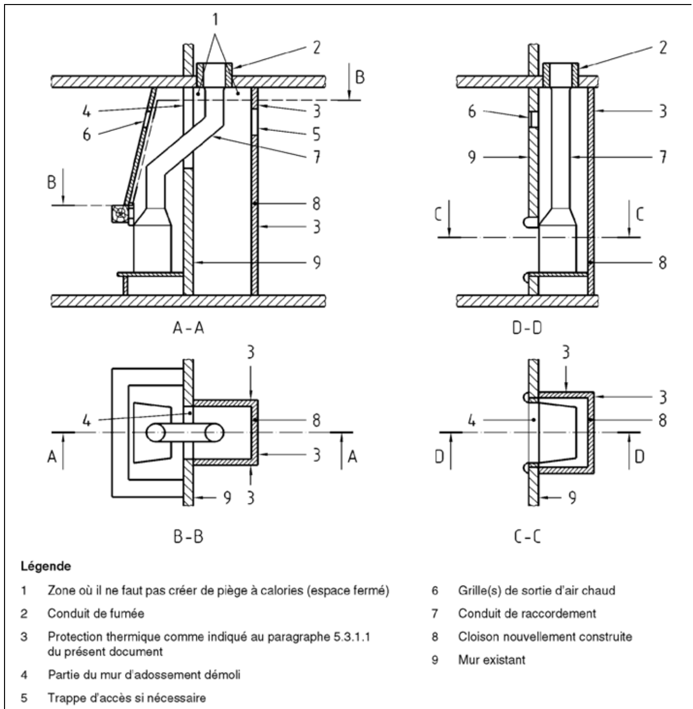
Figure 9 - Exemples de modification des caractéristiques des locaux dans le cas d'un conduit de fumée ne débouchant pas dans le local où est situé l'insert
